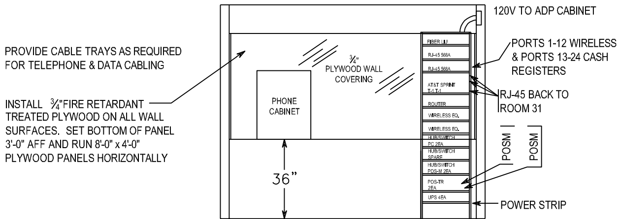
ELEVATION A-A
